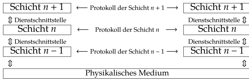
Bild 22.1: Protokolle und Dienstschnittstellen
