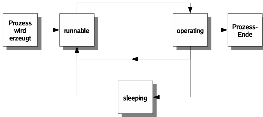
Bild 13.1: Verdeutlichung der Zusammenhänge zwischen den verschiedenen Prozesszuständen
