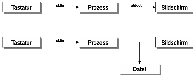
Bild 7.1: Standardkanäle unter Linux
