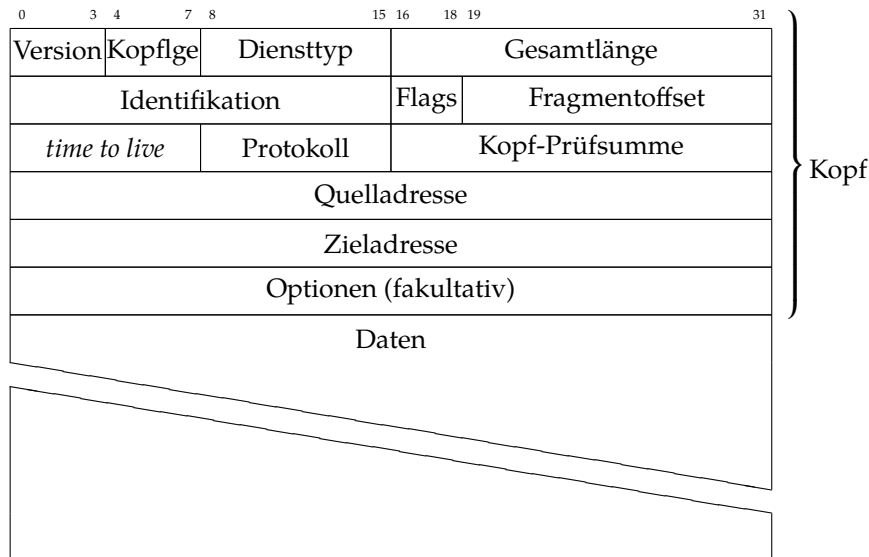
Bild 22.3: Aufbau eines IP-Datagramms. Jede Zeile entspricht 32 Bit.
