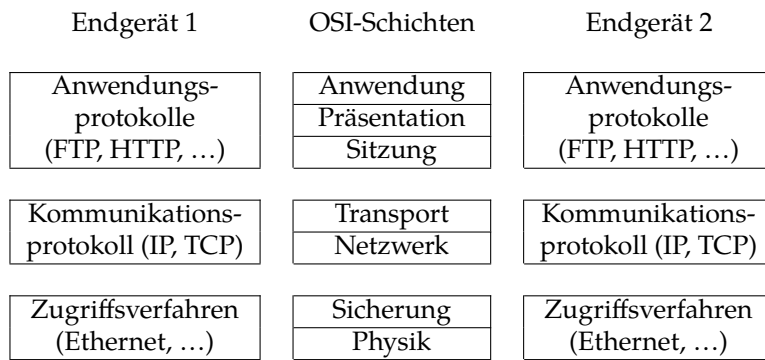
Bild 22.2: ISO/OSI-Referenzmodell
