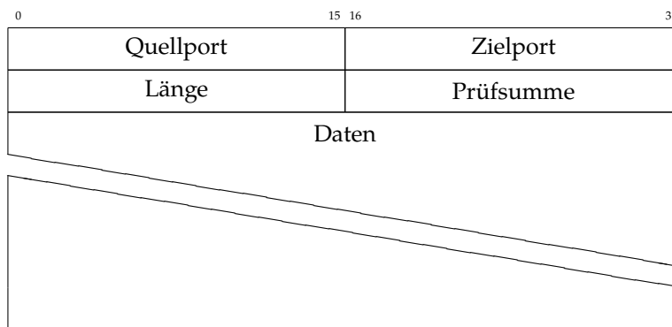
Bild 22.7: Aufbau eines UDP-Datagramms
