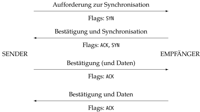
Bild 22.6: Aufbau einer TCP-Verbindung: Der Drei-Wege-Handshake
