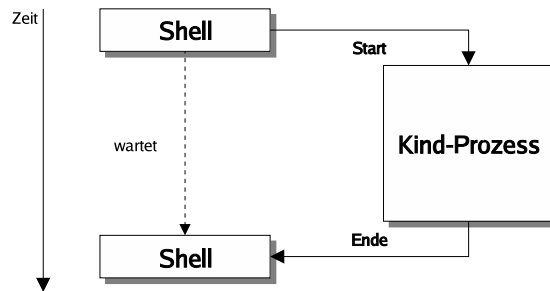
Bild 8.1: Die synchrone Arbeitsweise der Shell
