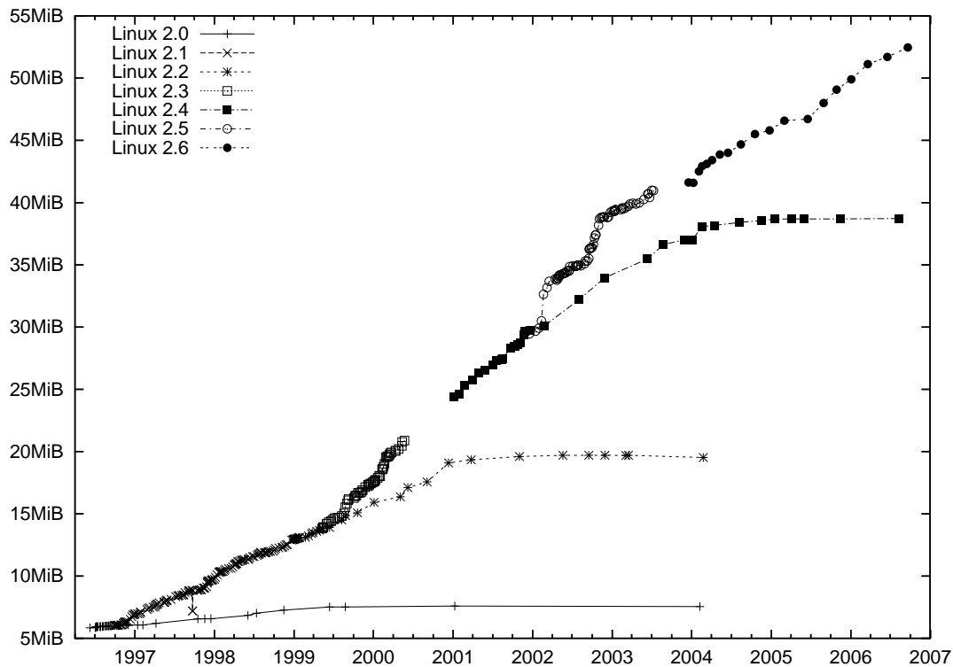
Bild 1.2: Die Weiterentwicklung von Linux, gemessen an der Größe von linux-*.tar.gz . Jede Marke entspricht einer Linux-Version. In den gut 10 Jahren von Linux 2.0 bis Linux 2.6.18 hat der Umfang des komprimierten Linux-Quellcodes sich nahezu verzehnfacht.
