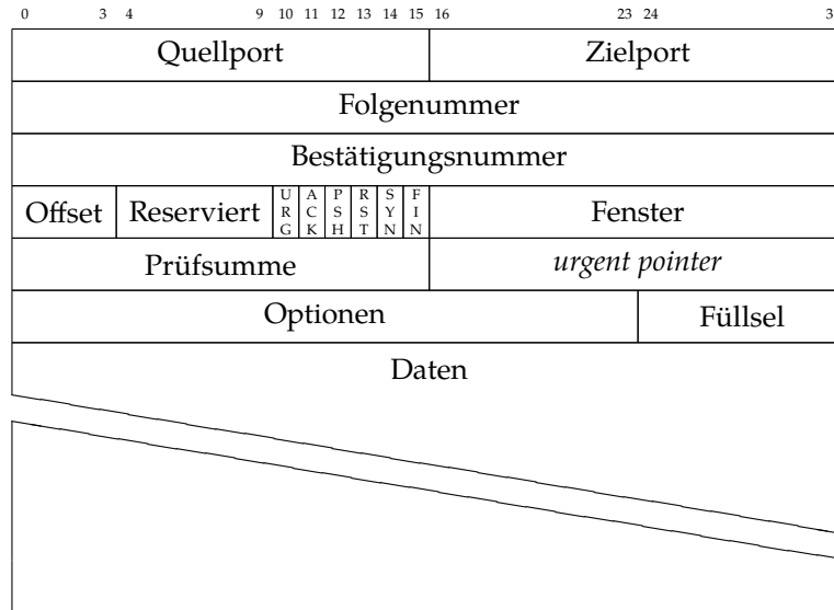
Bild 22.5: Aufbau eines TCP-Segments
